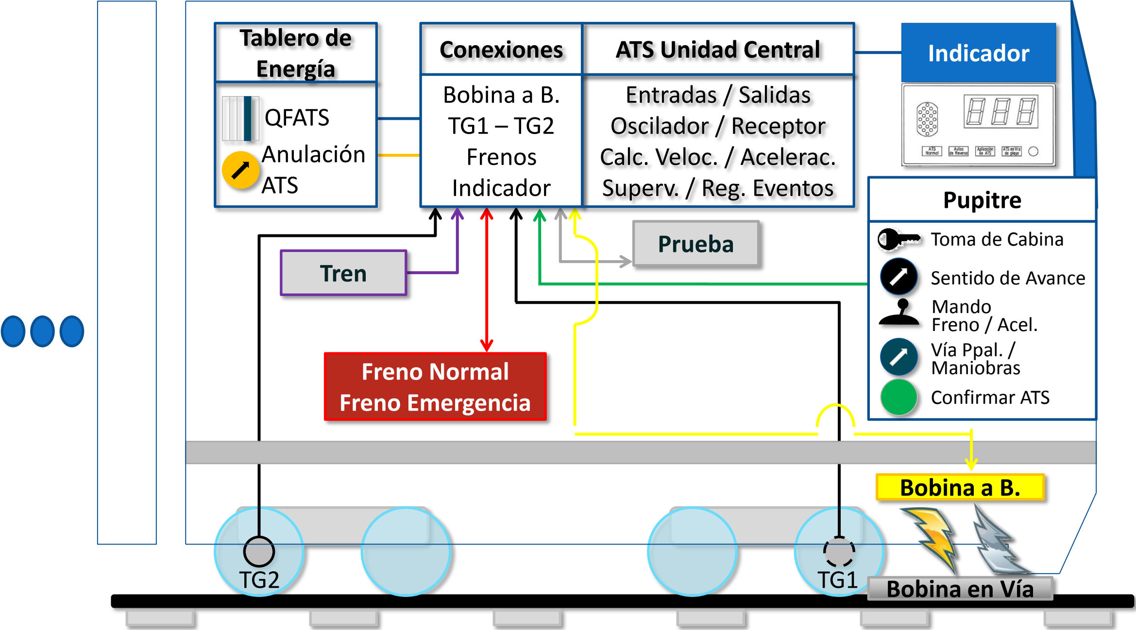
Esquema 01 DIAGRAMA EN BLOQUES ATS
