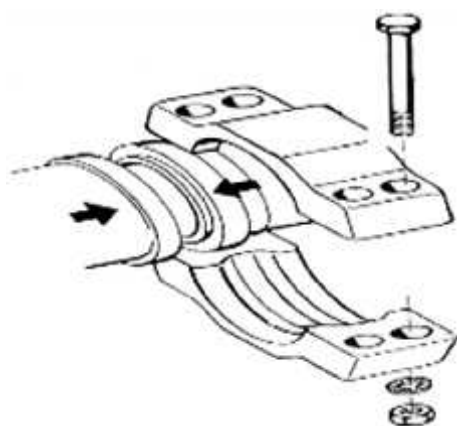
Figura 3. Montaje de un aro sujetador.
