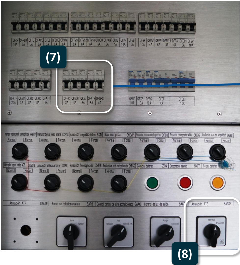
Imagen 05 TABLERO DE ENERGÍA – Cabina lateral derecho.
