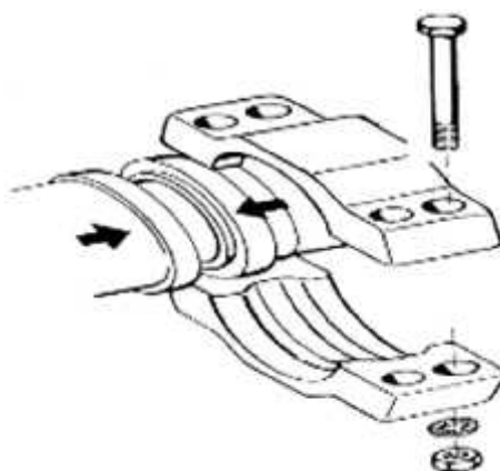
Figura 3. Montaje de un aro sujetador.
